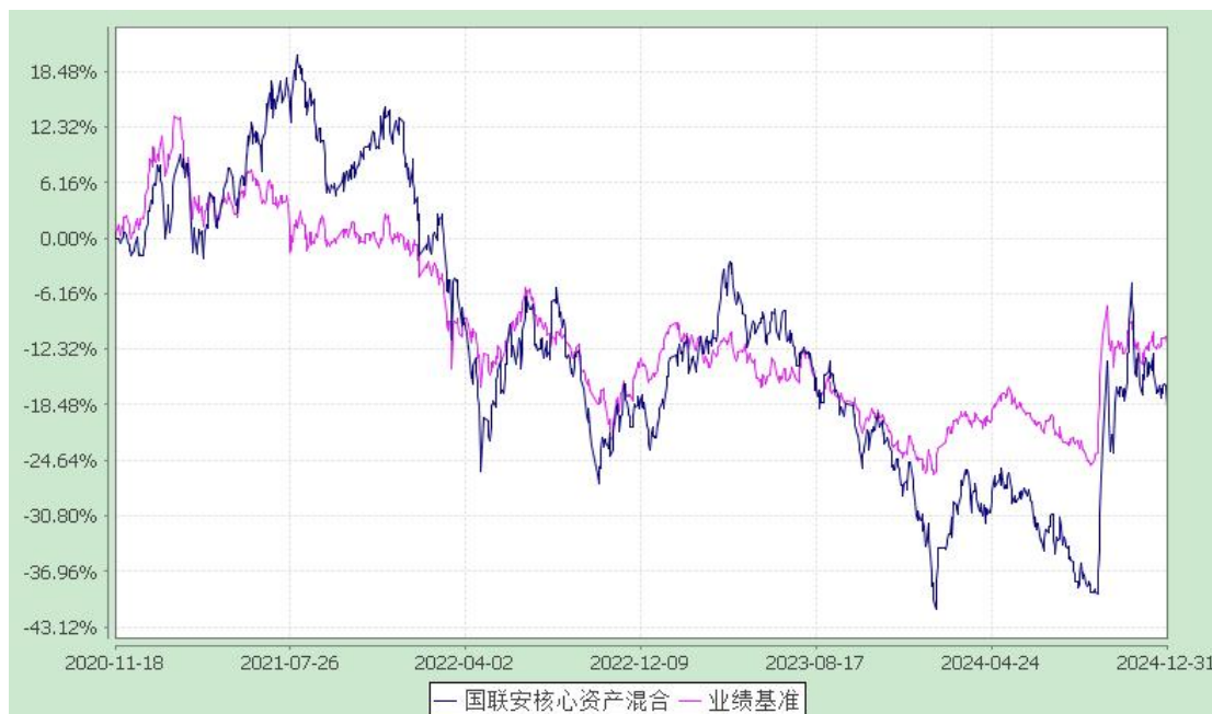
国联安核心资产策略混合型证券投资基金 累计净值增长率与业绩比较基准收益率历史走势对比图 (2020 年 11 月 18 日至 2024 年 12 月 31 日)
