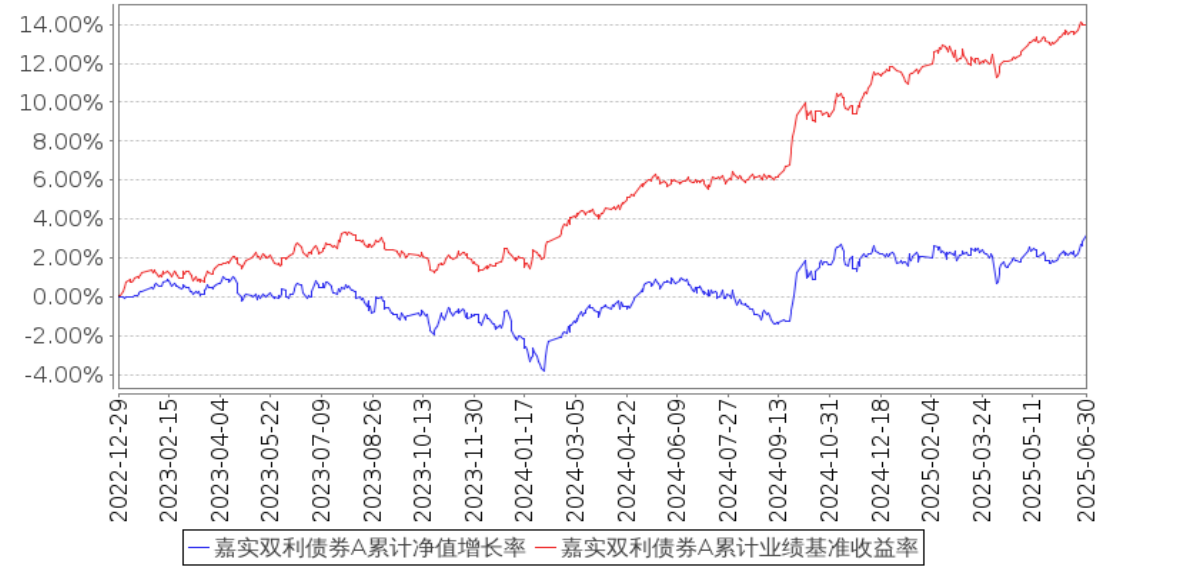
嘉实双利债券A累计净值增长率与同期业绩比较基准收益率的历史走势对比图 (2022年12月29日至2025年06月30日)
