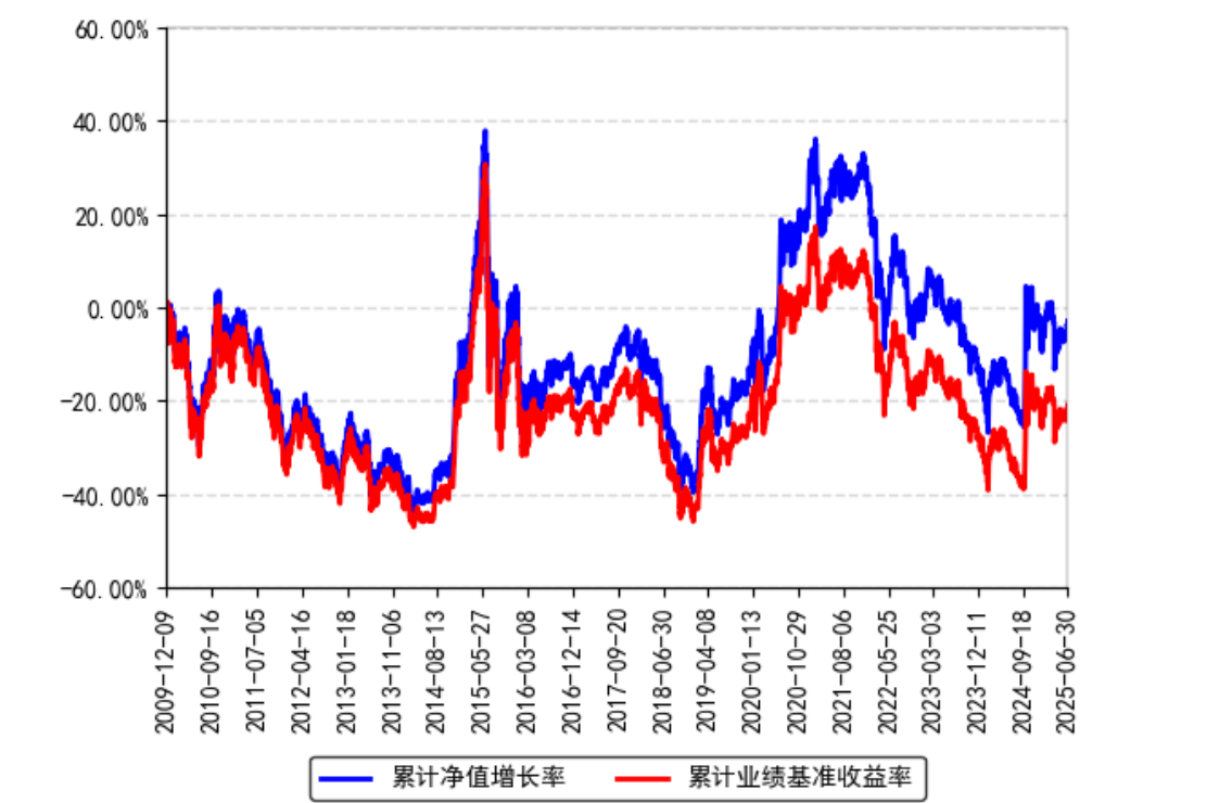
南方深证成份ETF联接A累计净值增长率与同期业绩比较基准收益率的历史走势对比图
