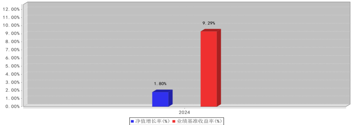
平安养老目标日期2050三年持有发起式（FOF）基金每年净值增长率与同期业绩比较基准收益率的对比图（2024年12月31日）
