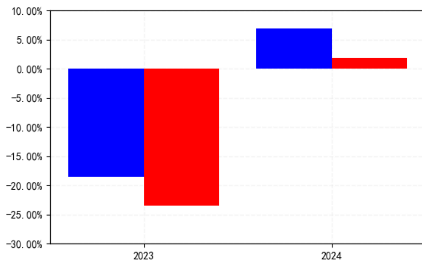
南方新材料股票发起A每年净值增长率与同期业绩比较基准收益率的对比图（2024年12月31日）
