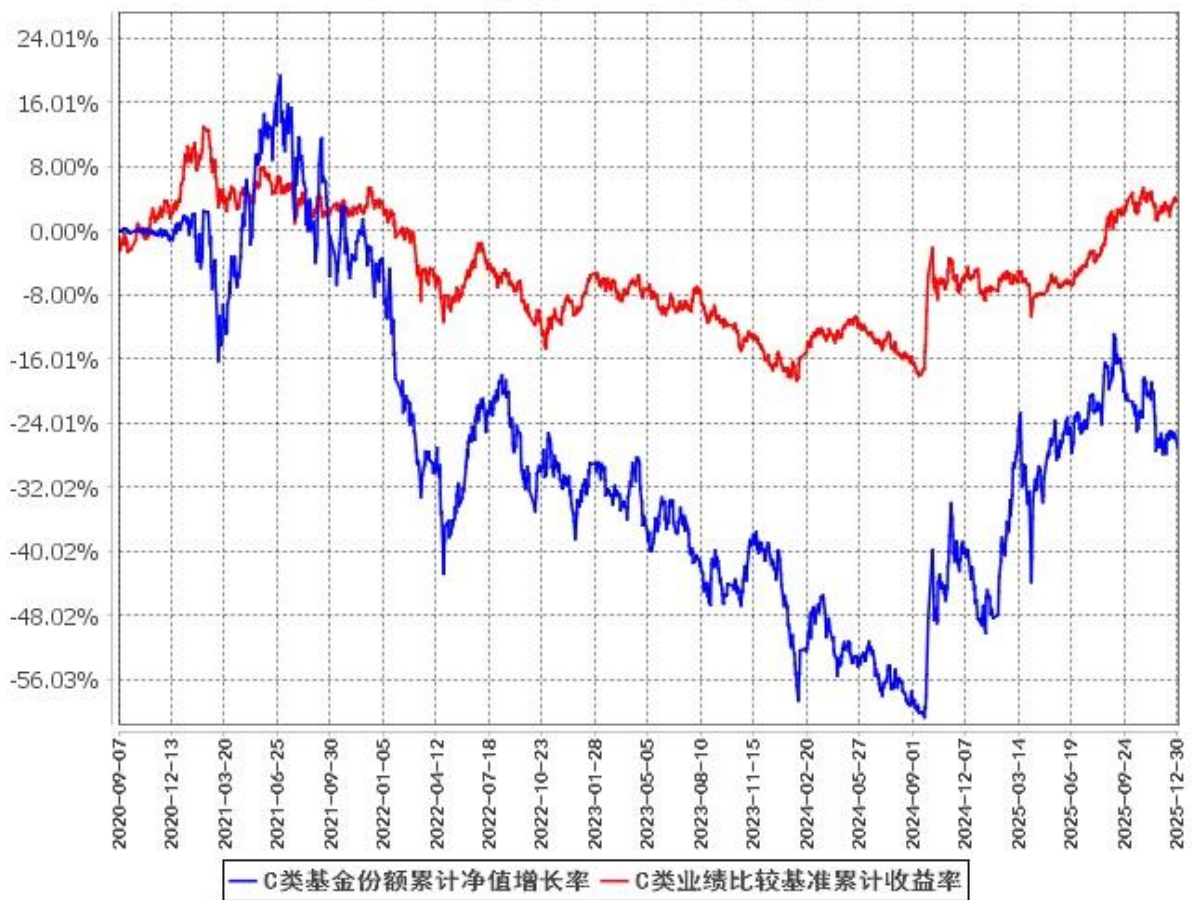
C类基金份额累计净值增长率与同期业绩比较基准收益率的历史走势对比图 (2020年9月7日至2025年12月31日)
