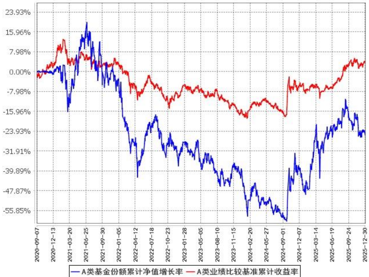
A类基金份额累计净值增长率与同期业绩比较基准收益率的历史走势对比图 (2020年9月7日至2025年12月31日)
