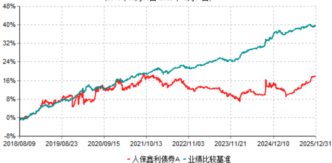
人保鑫利债券A累计净值增长率与业绩比较基准收益率历史走势对比图 (2018年08月09日-2025年12月31日)
