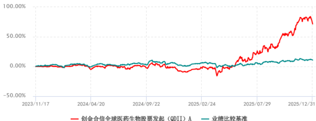
创金合信全球医药生物股票发起（QDII）A累计净值增长率与业绩比较基准收益率 历史走势对比图 (2023年11月17日-2025年12月31日)
