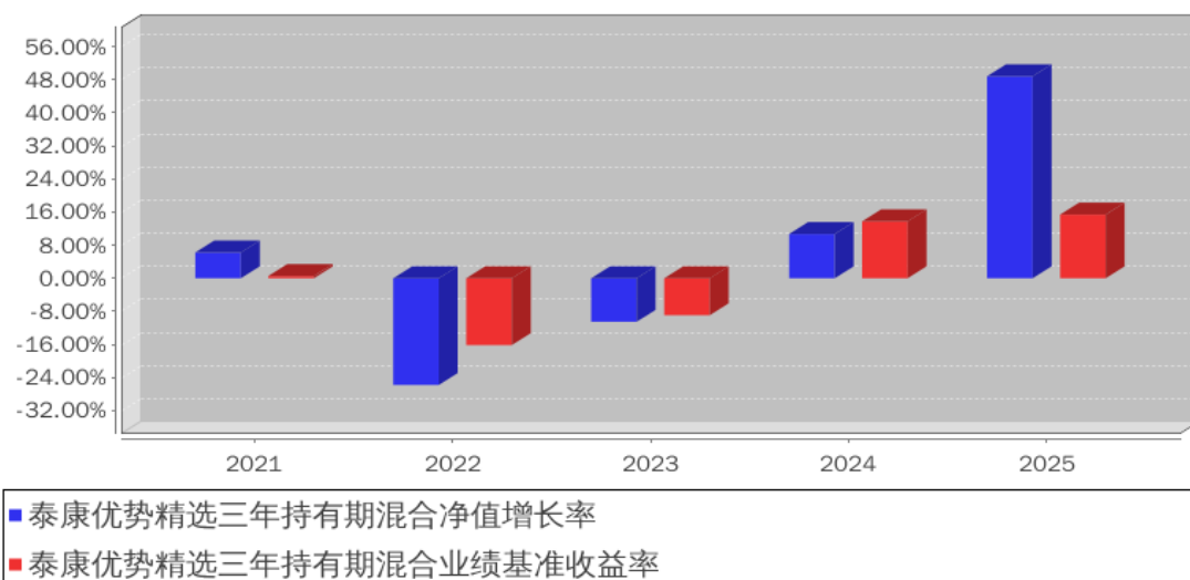
泰康优势精选三年持有期混合基金每年净值增长率与同期业绩比较基准收益率的对比图
