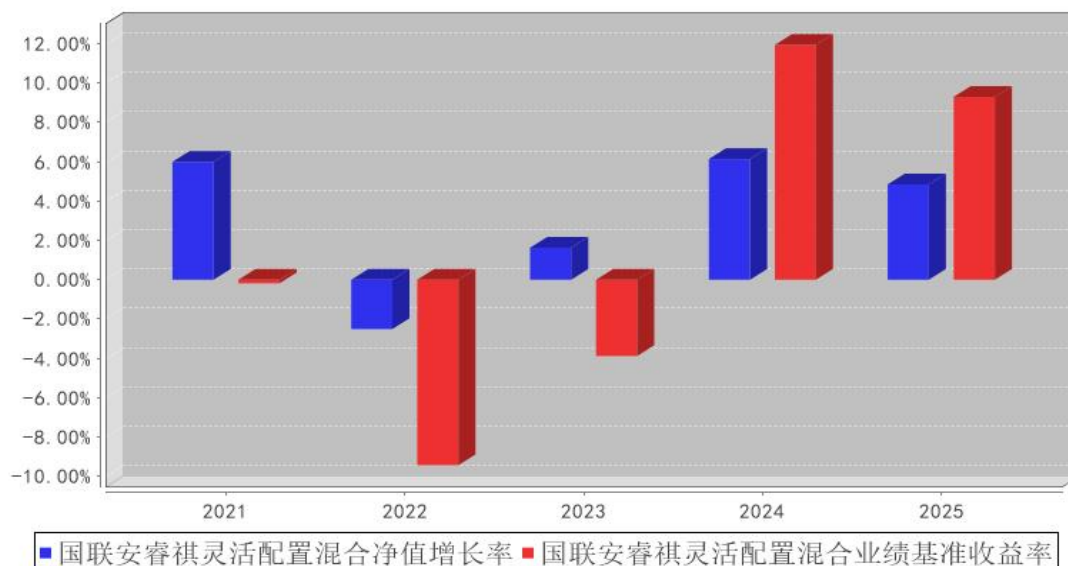
国联安睿祺灵活配置混合基金每年净值增长率与同期业绩比较基准收益率的对比图
