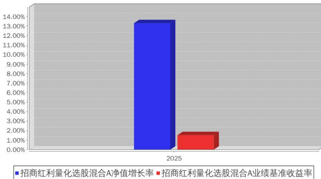
招商红利量化选股混合A基金每年净值增长率与同期业绩比较基准收益率的对比图
