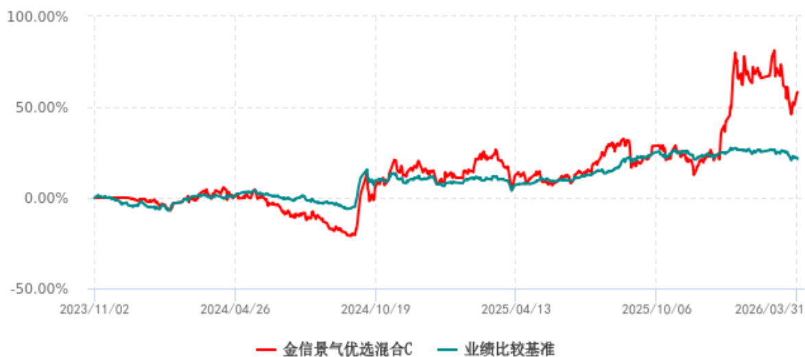
金信景气优选混合C累计净值增长率与业绩比较基准收益率历史走势对比图 (2023年11月02日-2026年03月31日)
