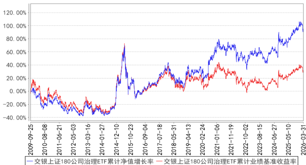
交银上证180公司治理ETF累计净值增长率与同期业绩比较基准收益率的历史走势图
