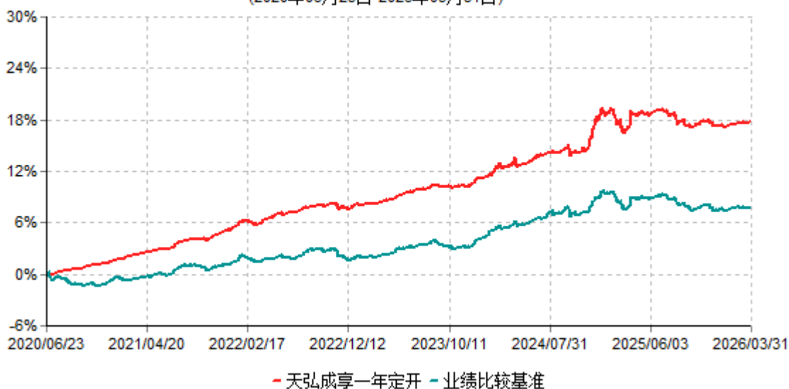
天弘成享一年定开累计净值增长率与业绩比较基准收益率历史走势对比图 (2020年06月23日-2026年03月31日)
