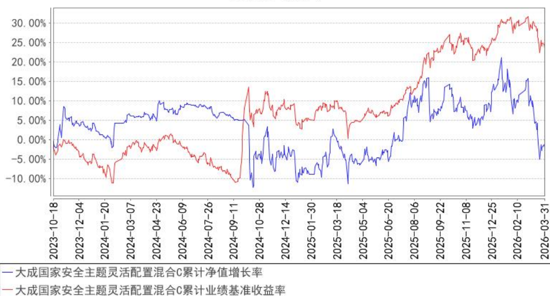
大成国家安全主题灵活配置混合C累计净值增长率与同期业绩比较基准收益率的历史走势对比图
