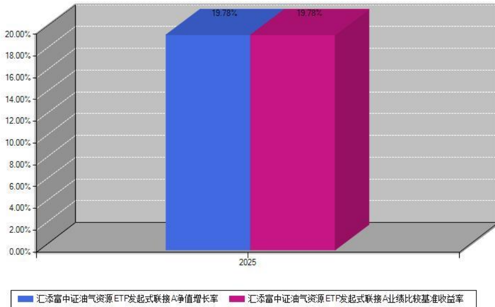
汇添富中证油气资源ETF发起式联接A每年净值增长率与同期业绩基准收益率对比图
