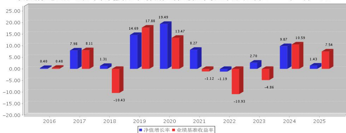
安信新优选混合C基金每年净值增长率与同期业绩比较基准收益率的对比图（2025年12月31日）
