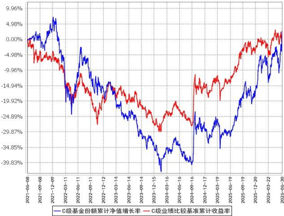
C级基金份额累计净值增长率与同期业绩比较基准收益率的历史走势对比图 (2021年6月8日至2026年6月30日)
