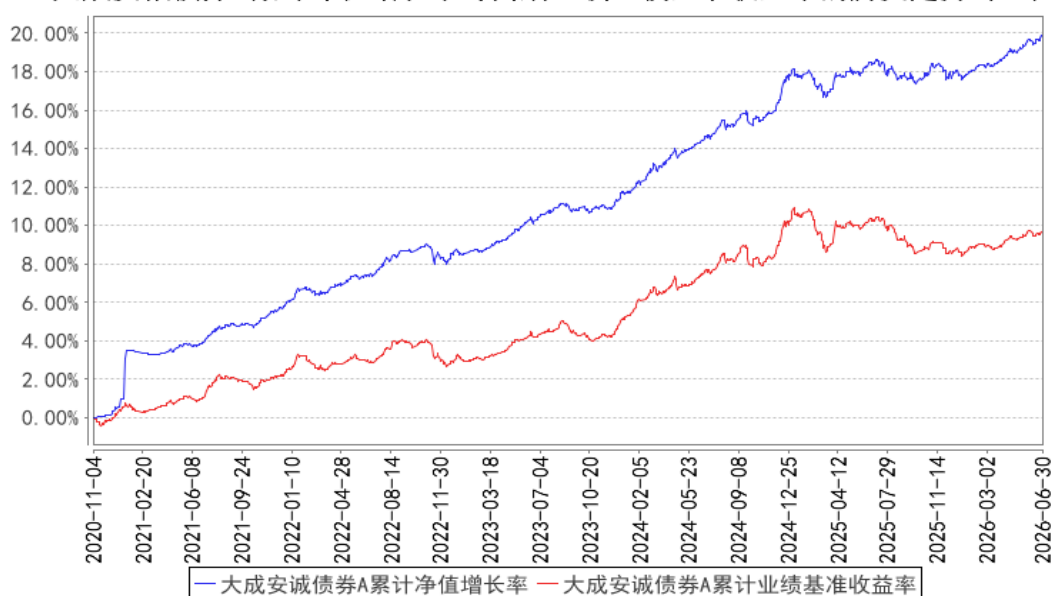
大成安诚债券A累计净值增长率与同期业绩比较基准收益率的历史走势对比图
