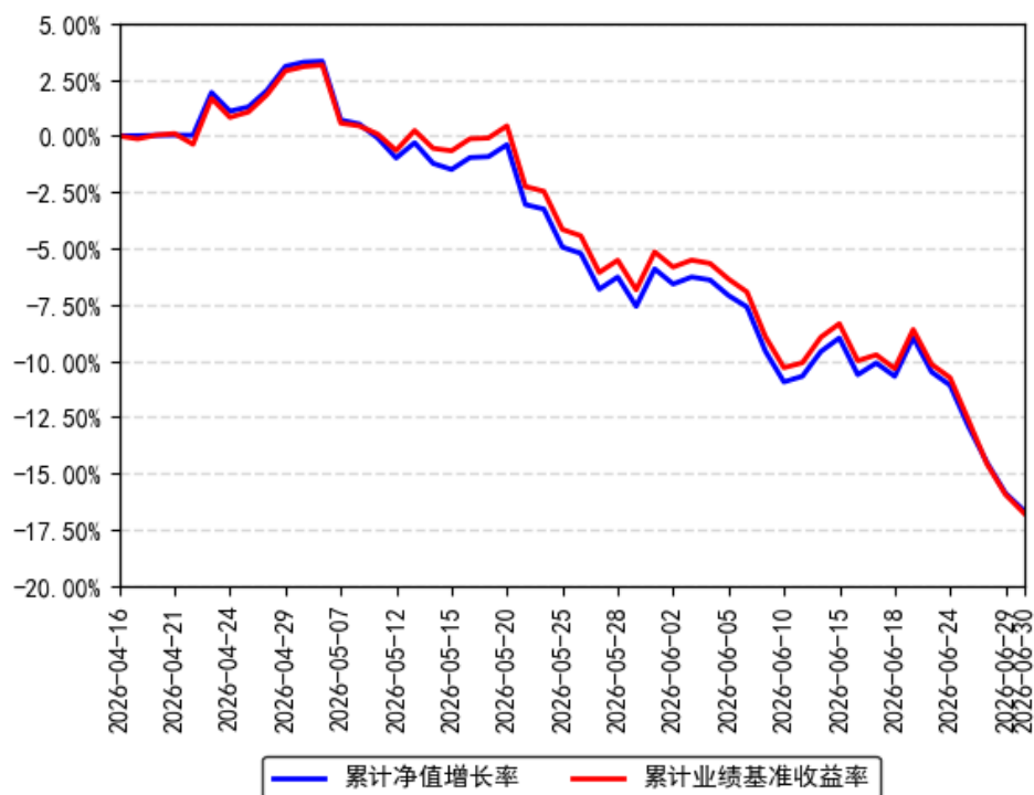
南方国证石油天然气ETF累计净值增长率与同期业绩比较基准收益率的历史走势对比图
