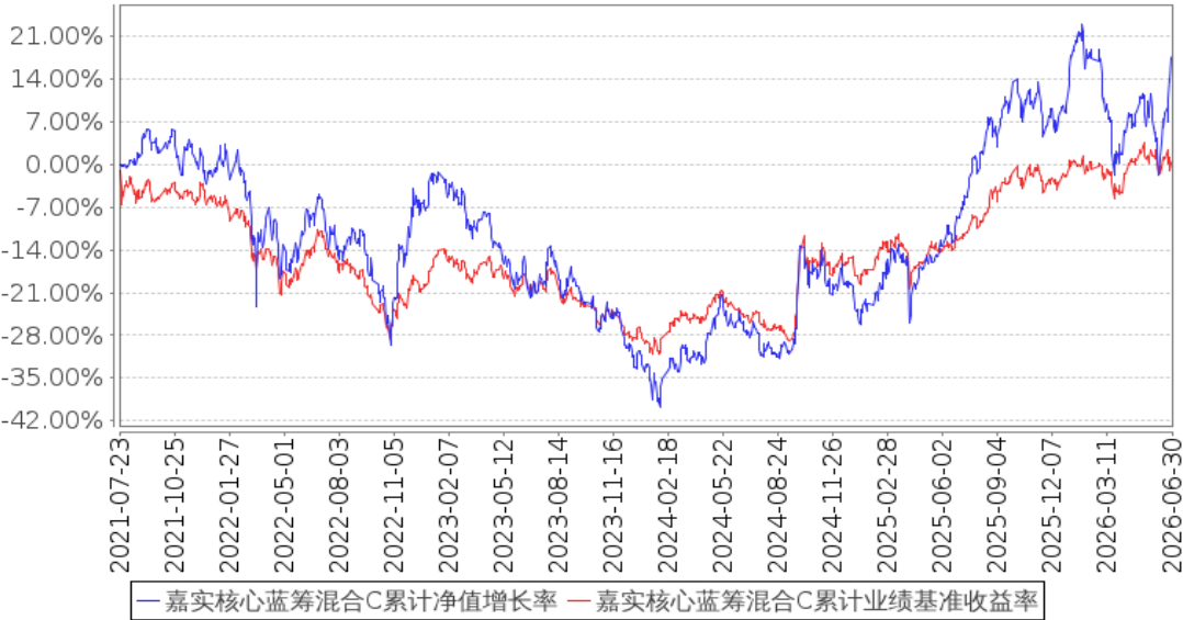
嘉实核心蓝筹混合C累计净值增长率与同期业绩比较基准收益率的历史走势对比图 (2021年07月23日至2026年06月30日)
