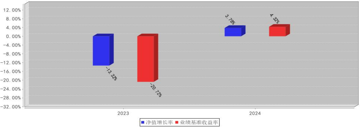
中航华证商飞高端制造产业指数发起C基金每年净值增长率与同期业绩比较基准收益率的对比图（2024年12月31日）
