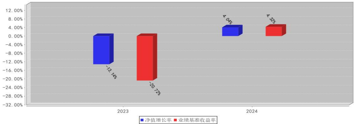
中航华证商飞高端制造产业指数发起A基金每年净值增长率与同期业绩比较基准收益率的对比图（2024年12月31日）
