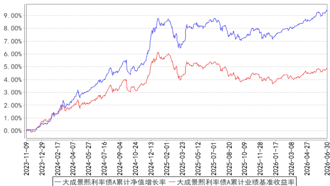
大成景熙利率债A累计净值增长率与同期业绩比较基准收益率的历史走势对比图
