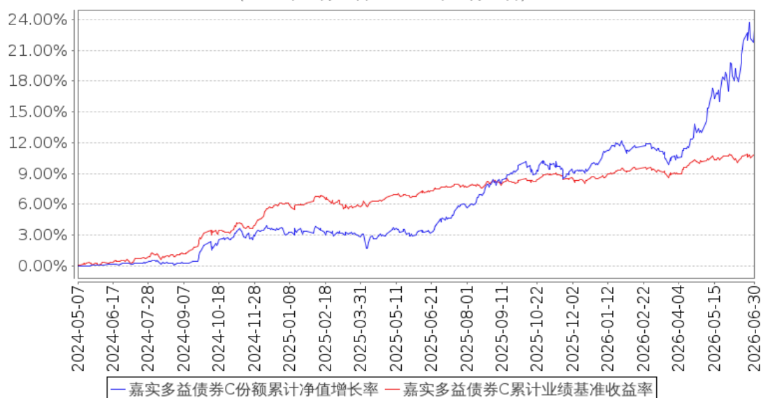
嘉实多益债券C份额累计净值增长率与同期业绩比较基准收益率的历史走势对比图
