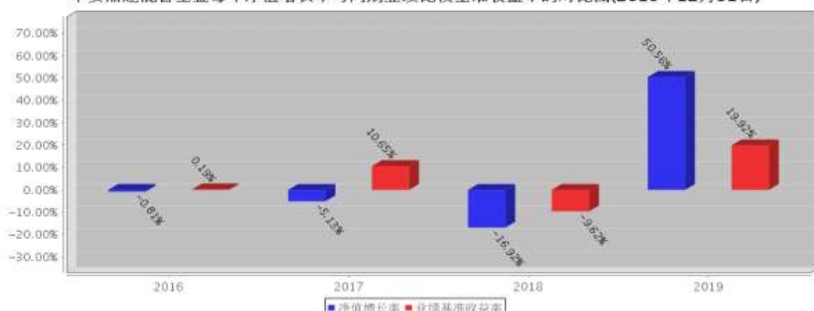
平安鼎越混合基金每年净值增长率与同期业绩比较基准收益率的对比图(2019年12月31日)
